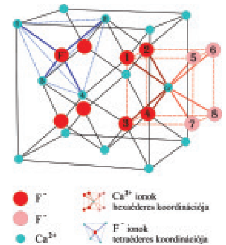
Az ionok elhelyezkedése a fluirit szerkezetét tükröző elemi cellán belül
